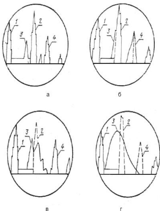
Рисунок Б.1 - Вид эхо-сигналов на экране дефектоскопа
